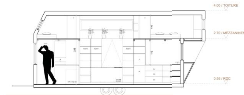
Coupe longitudinale
